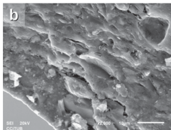
Fig.12. Micrografías de MEB a 2000X del individuo CER24. La escala gráfica representa 10 µm. a Resto de la matriz exhibiendo una alta concentración de pequeñas burbujas. b Exterior con un estado de sinterización de no vitrificación .
