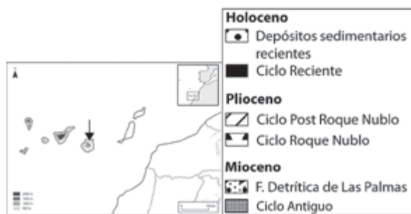
Fig. 1. Localización del yacimiento de La Cerera (LC, isla de Gran Canaria) y caracterización del entorno geológico (simplificado, Balcells et al. 1990).
